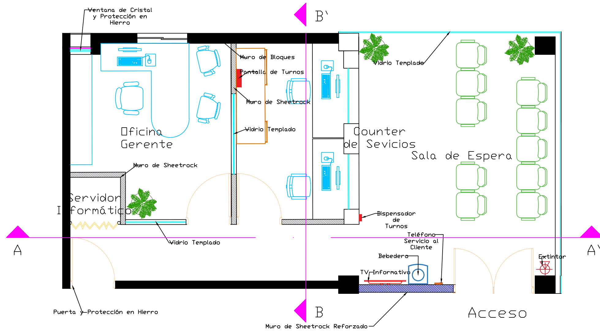
PLANTA AMUEBLADA PROYECTO :OFICINA LOCAL ADESS AREA = 48 m2
