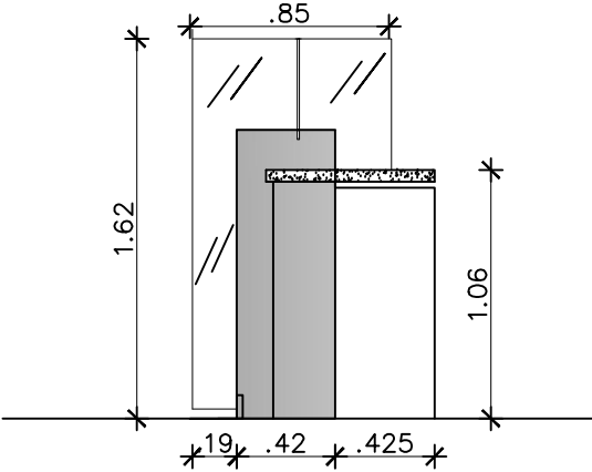
SECCION LATERAL
